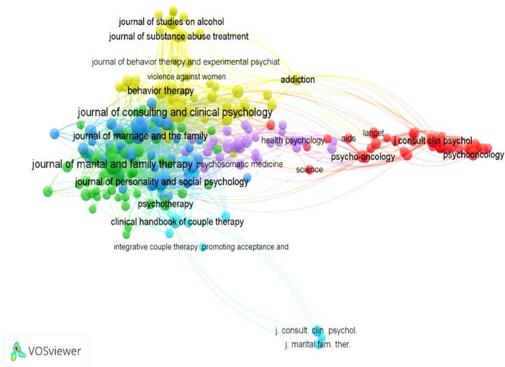
نمودار ۳. شبکه هم‌استنادی منابع
