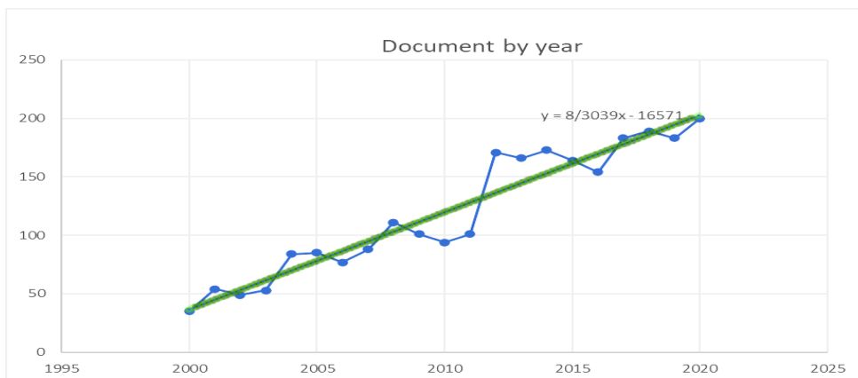
نمودار ۱. تعداد انتشار مدارک به ازای هر سال
