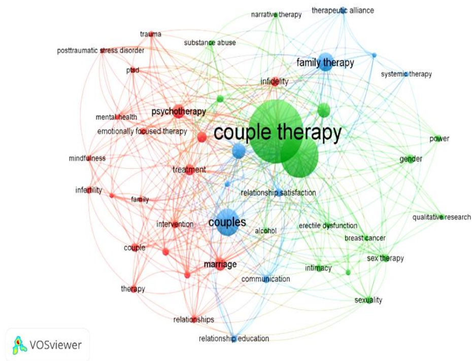
نمودار ۴: شبکه هم‌رخدادی کلمات کلیدی پرتکرار
